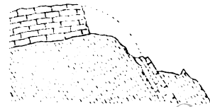
Fig. 12. Dem Gneiss parallele Einklemmung von Kalk bei der Eigerhöhle.
